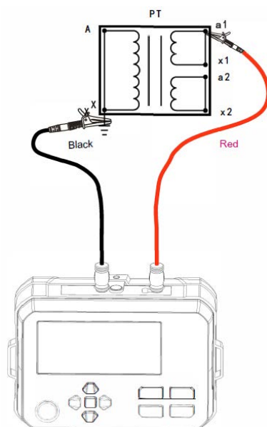
Obrázek 10.3 Schéma zapojení
