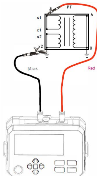
Obrázek 10.4 Schéma zapojení
