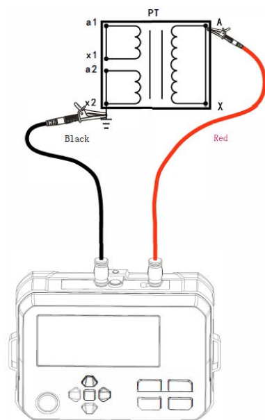
Obrázek 10.2 Schéma zapojení
