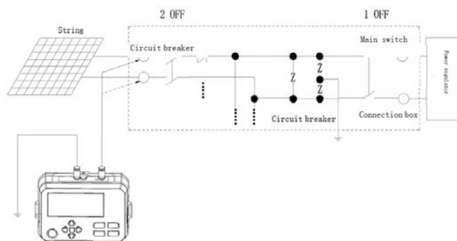
Obrázek 9.13 Fotovoltaická zařízení
