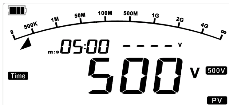
Figura 9.17 Misura dell'impostazione temporale del FV (interfaccia predefinita)
