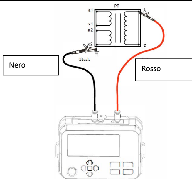
Figura 10.2 Diagramma di collegamento
