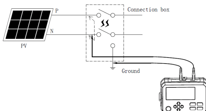
Figura 10.6 Misura tra P e N in stato di cortocircuito
