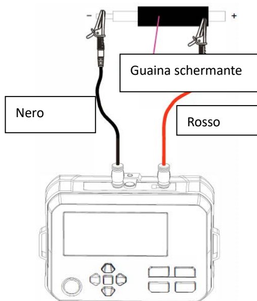
Figura 10.1 Misura convenzionale con metodo bifilare
