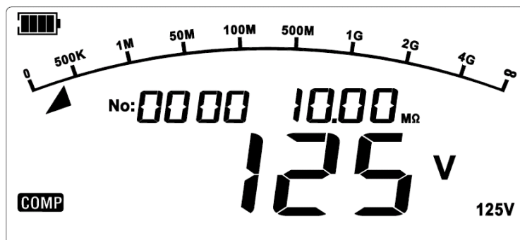
Figura 9.10 Misura della resistenza comparativa (interfaccia predefinita)
