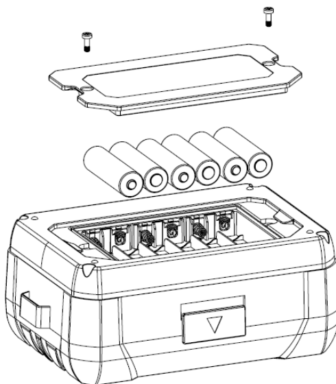
Figura 9.3 Installazione della batteria
