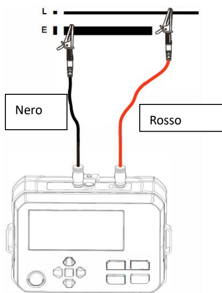
Figura 9.22 Collegamento della misura di tensione
