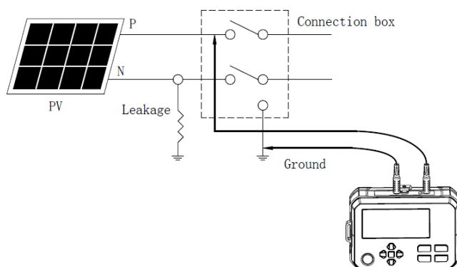
Figura 10.5 Misura tra P e N in stato di circuito aperto
