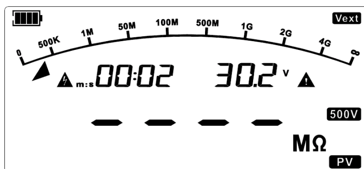
Figura 9.15 Rilevamento di una tensione esterna eccitata in modalità di misurazione della resistenza continua del FV
