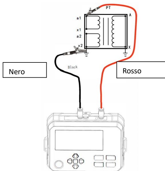
Figura 10.4 Diagramma di connessione
