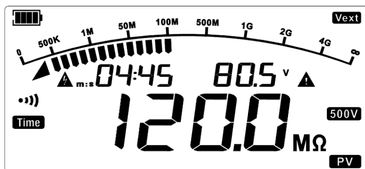
Figura 9.18 Durante la misurazione con timer fotovoltaico
