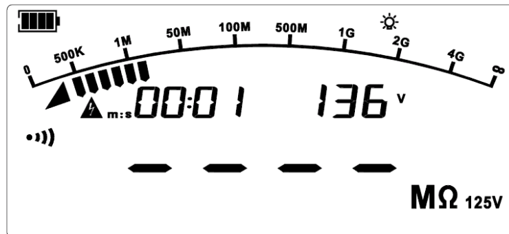
Figura 9.6 Durante la misurazione della resistenza continua
