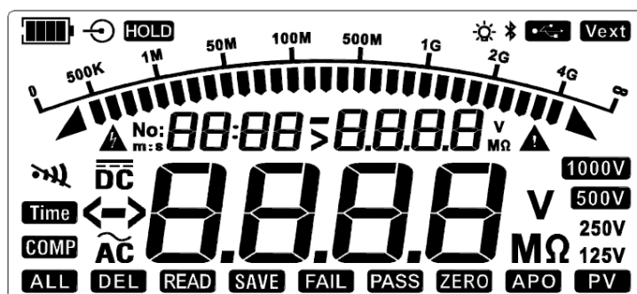
Figura 9.1 Tutti i segmenti visualizzati sul display LCD
