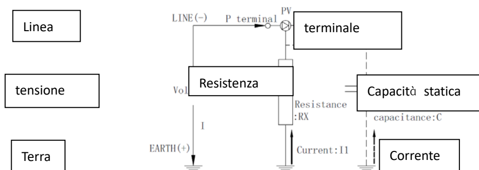
Figura 9.12 Principio di misurazione della resistenza fotovoltaica (PV)
