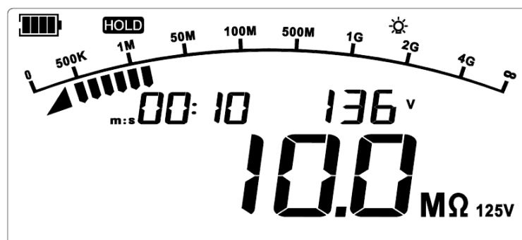
Figura 9.7 Interruzione della misurazione continua della resistenza
