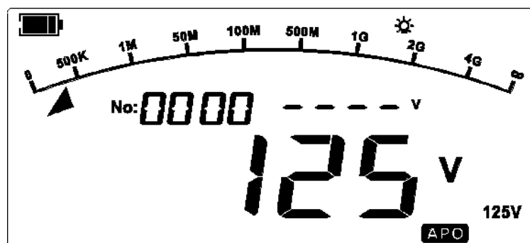
Figura 9.5 Misurazione continua della resistenza per impostazione predefinita dopo l'avvio
