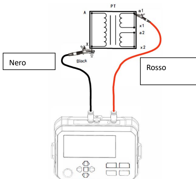
Figura 10.3 Diagramma di collegamento
