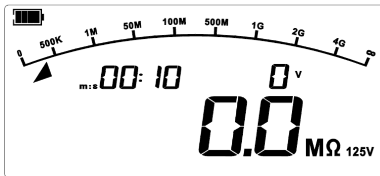
Figura 9.2 Conduttore di test in cortocircuito
