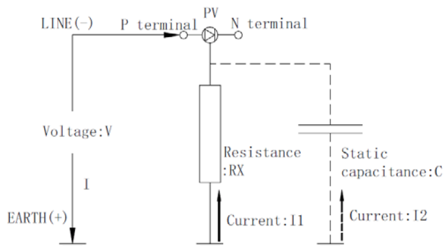
Rysunek 9.12 Zasada pomiaru rezystancji ogniw fotowoltaicznych (PV)
