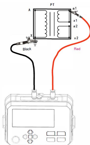
Rysunek 10.3 Schemat połączeń
